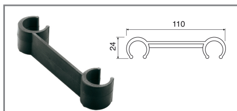
SISTEMA DI AGGANCIO LINKING SYSTEM
