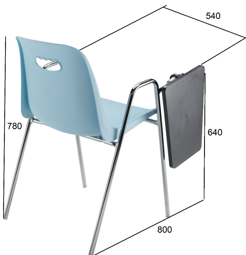
INGOMBRI MAX D18 CON TAVOLETTA
