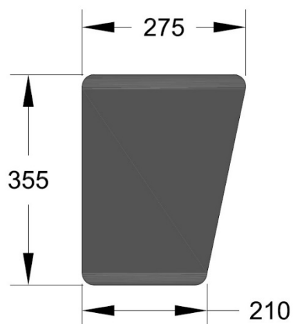
Dimensioni Tavoletta in ABS
