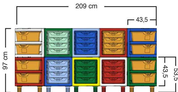
C002 3x2 + Cubeau angolare 3x2 + Corner Cubeau 3x2 + Cubeau angulaire
