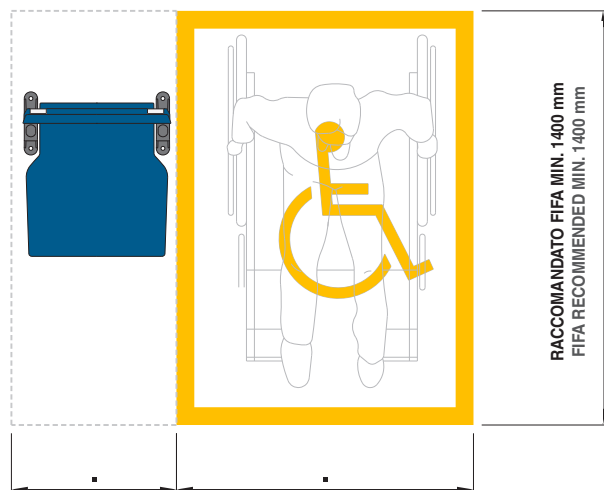
RACCOMANDATO FIFA MIN. 500 mm FIFA RECOMMENDED MIN. 500 mm RACCOMANDATO FIFA MIN. 900 mm FIFA RECOMMENDED MIN. 900 mm
