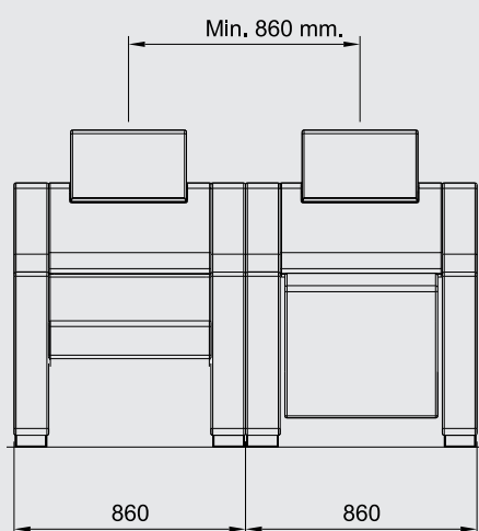
DOPPIO BRACCIOLO DOUBLE ARMREST
