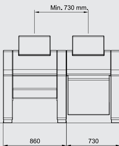
BRACCIOLO IN COMUNE SHARED ARMREST
