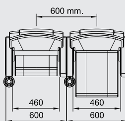
DOPPIO BRACCIOLO DOUBLE ARMREST
