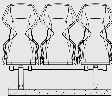
SU PANCA METALLICA ON METAL BENCH
