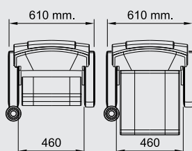
POLTRONA SINGOLA SINGLE ARMCHAIR
