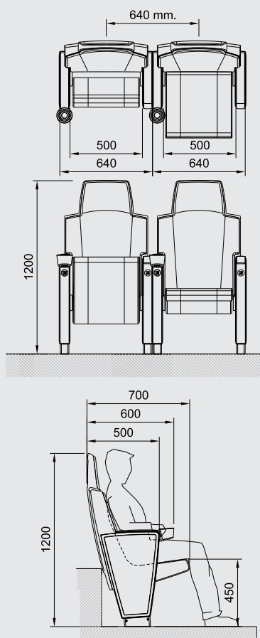
DOPPIO BRACCIOLO DOUBLE ARMREST
